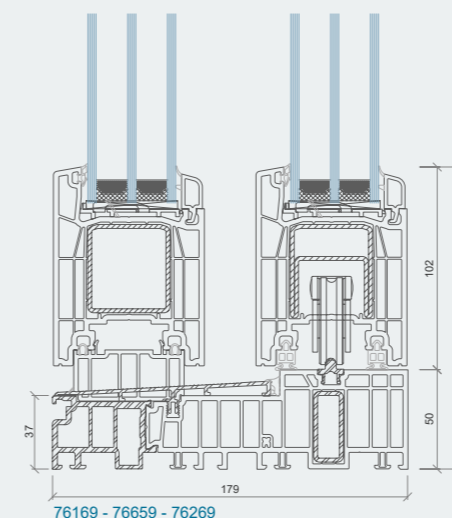
Secção PremiDoor76
